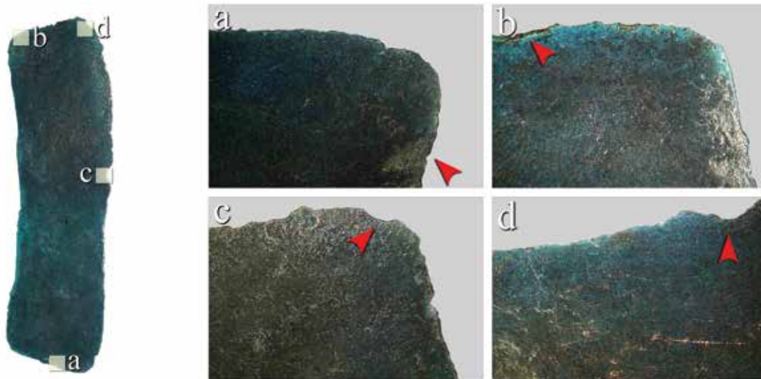
Ryc. 55. Makrostruktury brzytwy typu Biernatki War_9 z Wartosławia, gm. Wronki. Na zdjęciach widoczne są uszkodzenia mechaniczne i wynikające z procesów korozyjnych (pow. \times 3,5 ). Oprac. Łukasz Kowalski, Aldona Garbacz-Klempka, fot. Łukasz Kowalski
