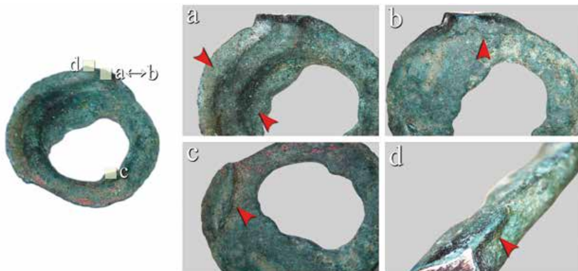
Ryc. 53. Makrostruktury kółka War_7 z Wartosławia, gm. Wronki. Na zdjęciach widoczne są (a) zalewki na płaszczyźnie podziału formy od strony wewnętrznej i zewnętrznej kółka oraz (c) ślady po układzie wlewowym (pow. \times 3,5 ). Oprac. Łukasz Kowalski, Aldona Garbacz-Klempka, fot. Łukasz Kowalski
