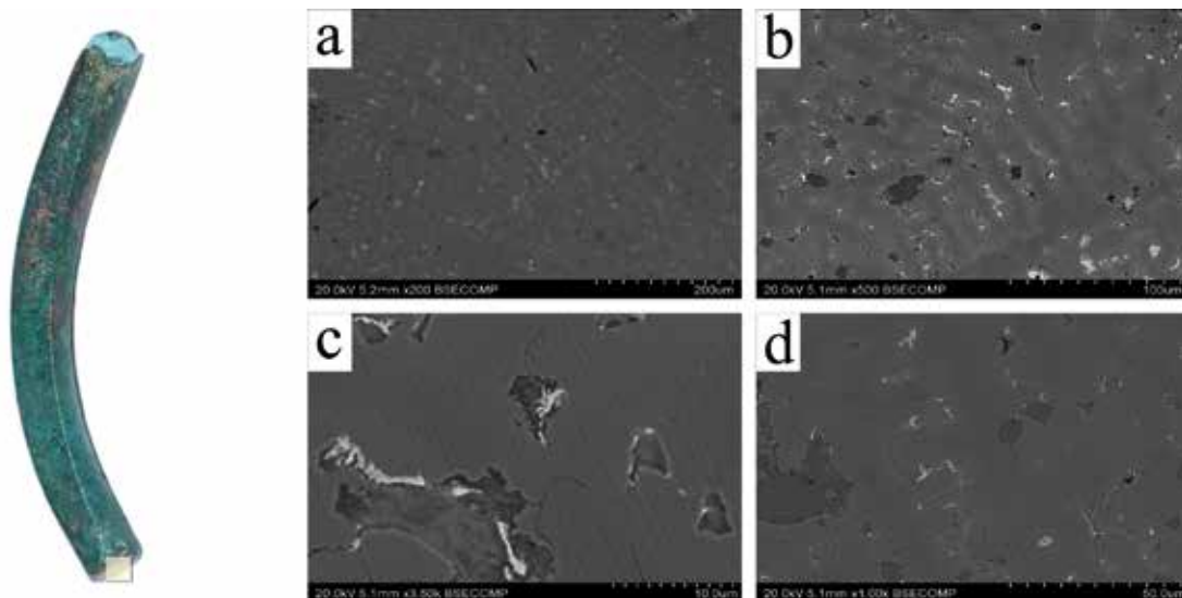
Ryc. 49. Obrazy BSE mikrostruktur pręcika War_8 z Wartosławia, gm. Wronki. Widoczna jest struktura dendrytyczna roztworu stałego niklu i arsenu w miedzi. W przestrzeniach pomiędzy dendrytami widoczne są fazy międzymetaliczne zawierające miedź, arsen i antymon oraz małe białe wydzielania ołowiu. Struktura dendrytyczna dowodzi, że prętek był odlewany, a zniekształcenie faz międzymetalicznych, dowodzi dodatkowo że przedmiot był przerabiany plastycznie; (a) pow. \times 200 , (b) pow. \times 500 , (d) pow. \times 1000 , (c) pow. \times 3500 . Oprac. Łukasz Kowalski, Aldona Garbacz-Klempka, fot. Łukasz Kowalski
