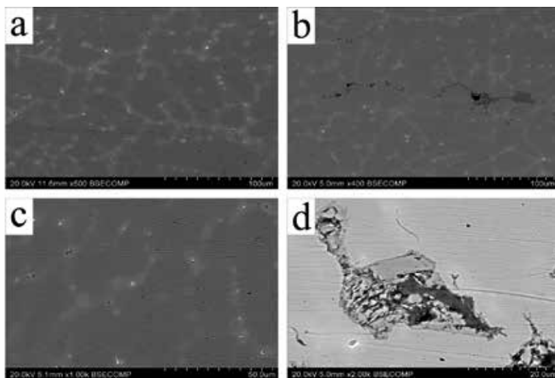
Ryc. 48. Obrazy BSE mikrostruktur kółka War_7 z Wartosławia, gm. Wronki. Widoczne są (a, b, c) wydzielania faz międzymetalicznych składników niskotopliwych: srebra, antymonu i ołowiu w przestrzeniach międzydendrycznych oraz (d) ogniska korozji; (a) pow. \times 500 , (d) pow. \times 1000 , (c) pow. \times 2500 , (b) pow. \times 4000 . Oprac. Łukasz Kowalski, Aldona Garbacz-Klempka, fot. Łukasz Kowalski
