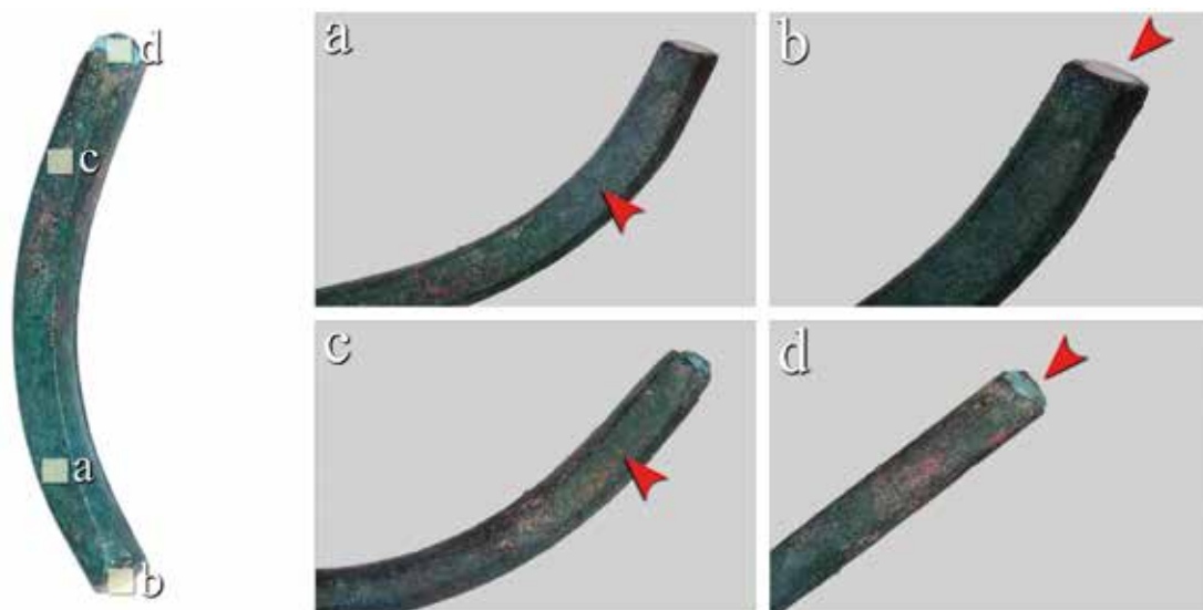
Ryc. 54. Makrostruktury pręcika War_8 z Wartosławia, gm. Wronki. Na zdjęciach widoczny jest pręt po odlaniu i po przeróbce plastycznej (pow. \times 3,5 ). Oprac. Łukasz Kowalski, Aldona Garbacz-Klempka, fot. Łukasz Kowalski
