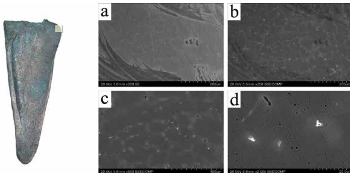
Ryc. 46. Obrazy BSE mikrostruktur fragmentu sierpa War_1 z Wartosławia, gm. Wronki. Na tle ciemnych dendrytów roztworu stałego cyny i niklu w miedzi widoczne są w przestrzeniach międzydendrytycznych jaśniejsze wydzielania eutektoidu zawierającego miedź i cynę (b i c) oraz białe wydzielania ołowiu (d); (a, b) pow. \times 200 , (c) pow. \times 500 , (d) pow. \times 2000 . Oprac. Łukasz Kowalski, Aldona Garbacz-Klempka, fot. Łukasz Kowalski
