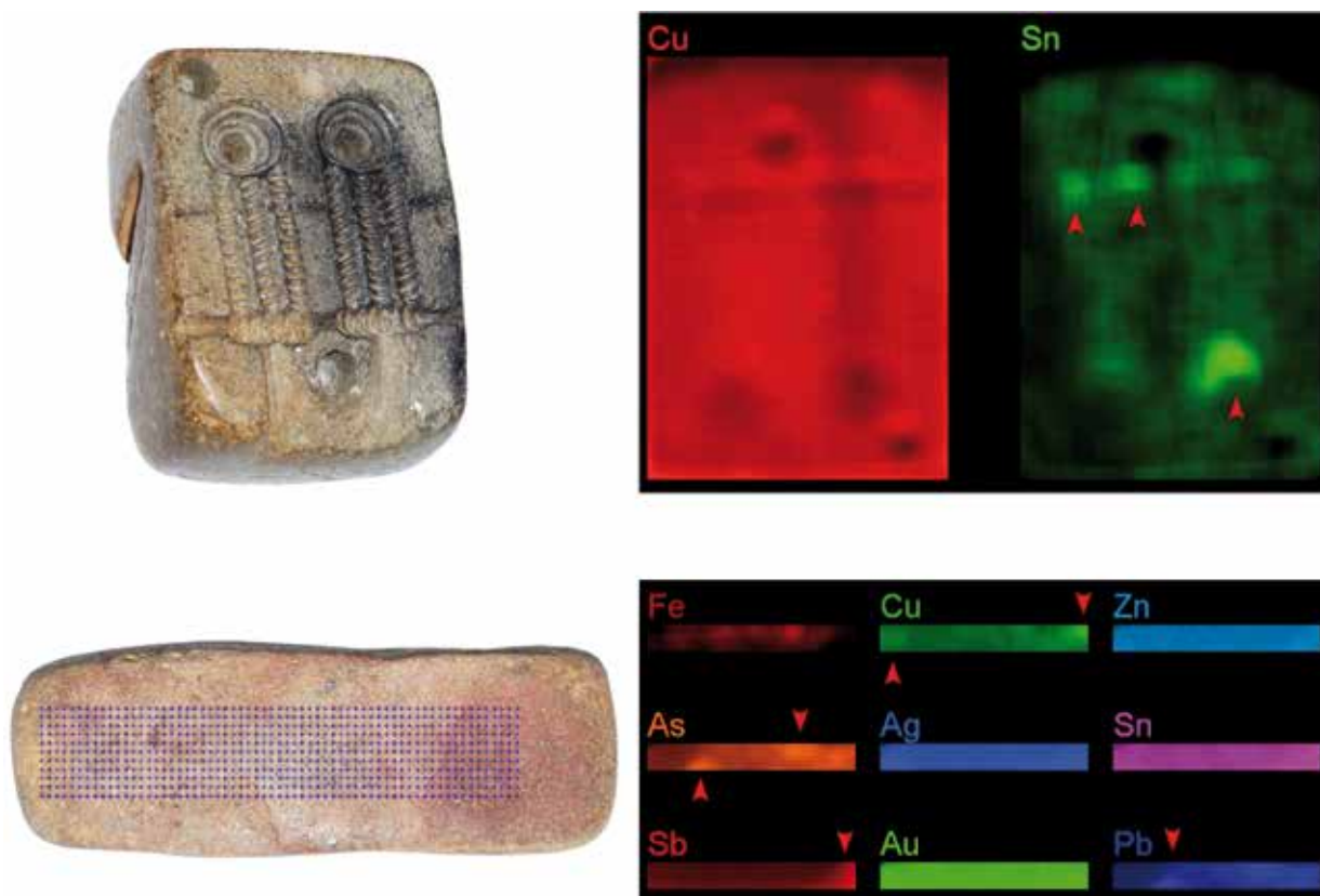
Ryc. 45. Rozkład pierwiastków metalicznych na powierzchniach półówki formy odlewniczej War_13 i gładzika War_16 z Wartosławia, gm. Wronki. Oprac. Łukasz Kowalski, Aldona Garbacz-Klempka, fot. Łukasz Kowalski
