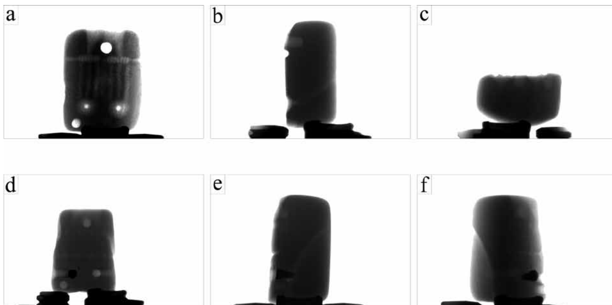
Ryc. 58. Obrazy rentgenowskie kamiennej formy odlewniczej z Wartosławia gm. Wronki. Widoczne są (a) wnętrza formy wraz z układem wlewowym dwukanałowym, (d) gniazdo rdzennika, (d) kanały odpowietrzające oraz (a, d) otwory na kołki centrujące. Czytelny jest (d-f) metaliczny czop blokujący kanał formy. Oprac. Łukasz Kowalski, Aldona Garbacz-Klempka, fot. Łukasz Kowalski
