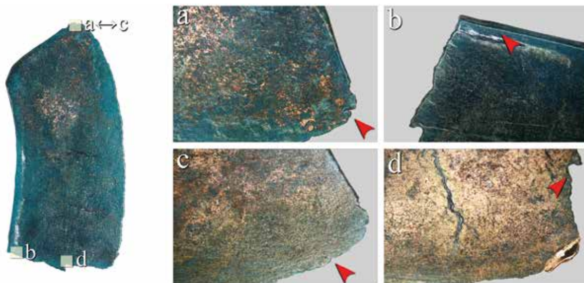
Ryc. 52. Makrostruktury brzytwy typu Biernatki War_6 z Wartosławia, gm. Wronki. Na zdjęciach widoczne są (d) uszkodzenia mechaniczne w postaci pęknięć prawdopodobnie wzdłuż granic ziaren oraz (a, c) wyszczerbienia krawędzi (pow. \times 3,5 ). Oprac. Łukasz Kowalski, Aldona Garbacz-Klempka, fot. Łukasz Kowalski
