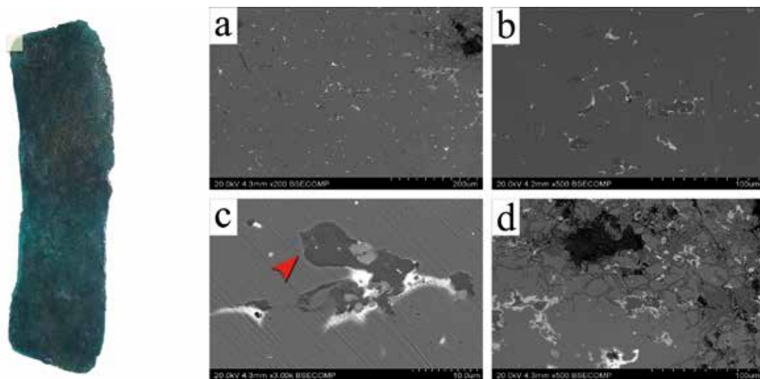
Ryc. 50. Obrazy BSE mikrostruktur brzytwy War_9 z Wartosławia, gm. Wronki. Osnowę stopu tworzy miedź z cyną i arsenem, a w niej dość liczne i rozległe (a) białe skupiska ołowiu, który wykazuje z miedzią brak rozpuszczalności. Widoczne są (d) granice ziaren, a na granicach produkty korozji o charakterze tlenkowym. Lokalnie występują (c) wydzielania siarczków; (a) pow. \times 200 , (b, d) pow. \times 500 , (c) pow. \times 3000 . Oprac. Łukasz Kowalski, Aldona Garbacz-Klempka, fot. Łukasz Kowalski
