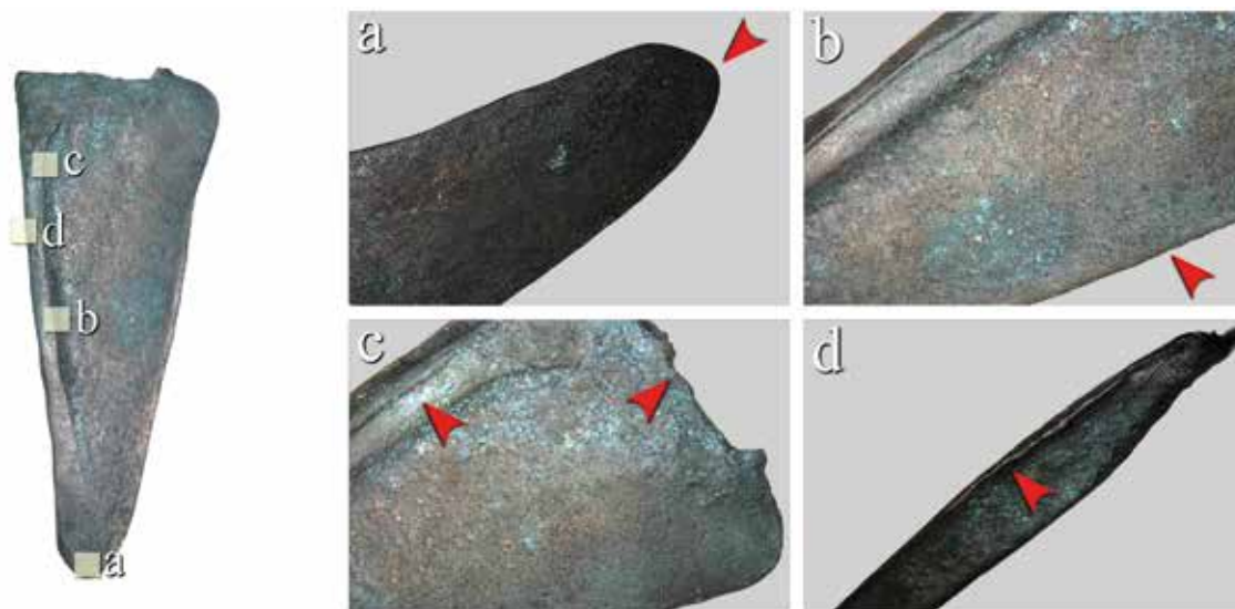
Ryc. 51. Makrostruktury fragmentu sierpa War_1 z Wartosławia, gm. Wronki. Na zdjęciach widoczne są powierzchnie pozbawione wad odlewniczych, które nie były poddawane przeróbce plastycznej (pow. \times 3,5 ). Oprac. Łukasz Kowalski, Aldona Garbacz-Klempka, fot. Łukasz Kowalski
