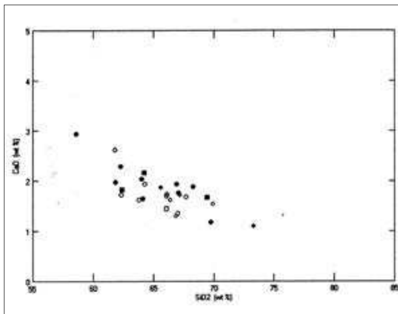
Ryc. 2. Zawada, stan. 1, gm. Zielona Góra. Diagram \text{SiO}_2 -CaO
