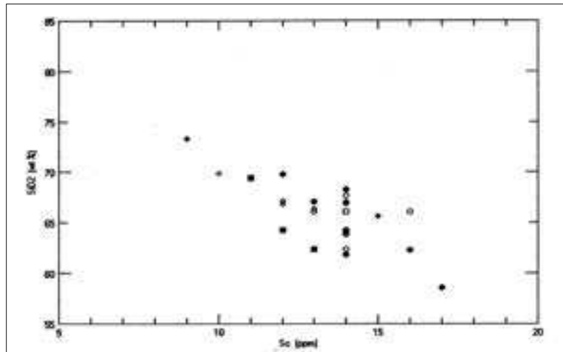
Ryc. 20. Zawada, stan. 1, gm. Zielona Góra. Diagram Sc-SiO 2 1
