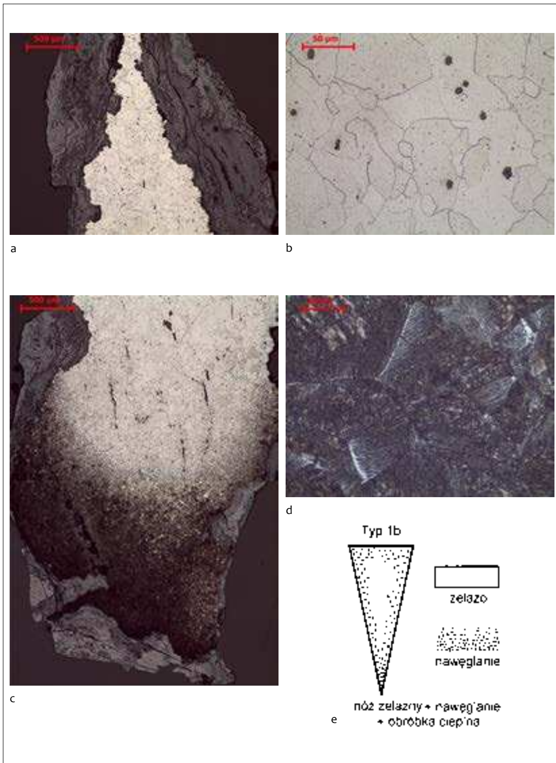
Ryc. 7. Zawada, stan. 1, gm. Zielona Góra. Fragment noża żelaznego, nr kat. 1992: 48, próbka nr 1: a – warstwienia produktów korozji przy powierzchniach noża w obszarze 2; b – ferryt oraz wtrącenia żużla w obszarze 2; c – tylec noża, obszar 3; d – mikrostruktura w tylcu noża: martenzyt odpuszczony, bainit, troostyt oraz ferryt, obszar 3; e – prawdopodobna technologia wykonania noża typ 1b
