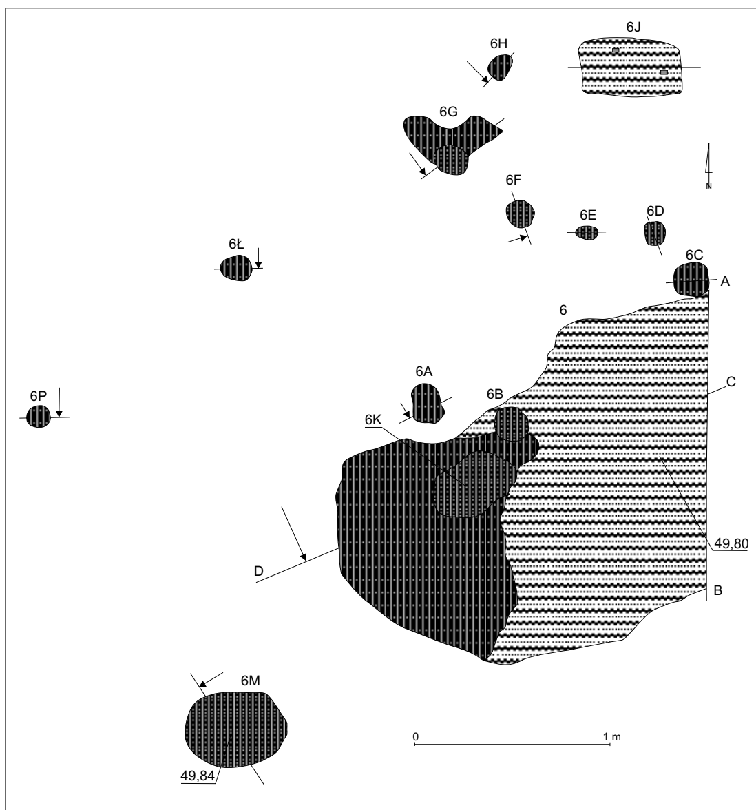
Ryc. 8. Zawada, stan. 1, pow. zielonogórski. Rzuty poziome obiektu 6 i związanych z nim dołków postępujących. Rys. S. Kałagata, oprac. B. Gruszka
