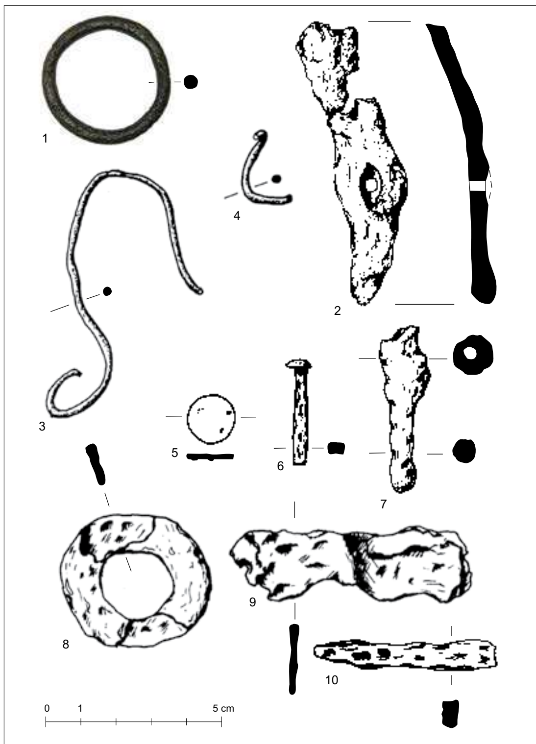
Ryc. 2. Zawada, stan. 1, gm. Zielona Góra. Zabytki odkryte podczas badań. 1 – krępulec wędzidła, 2 – fragment podkowy, 3, 4 – fragmenty drutów, 5 – guzik lub apilkacja, 7 – tuleja grotu strzały, 8 – podkładka?, 9 – fragment blachy. 1-2, 4, 6-9 – żelazo, 3, 5 – brąz. Rys. S. Kałagate, fot. A. Michalak
