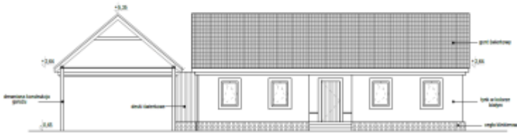
RYS. 5. ELEWACJA PÓŁNOCNA SKALA 1:100
