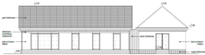
RYS. 4. ELEWACJA POŁUDNIOWA SKALA 1:100
