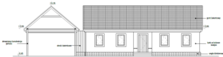
RYS. 5. ELEWACJA PÓŁNOCNA SKALA 1:100
